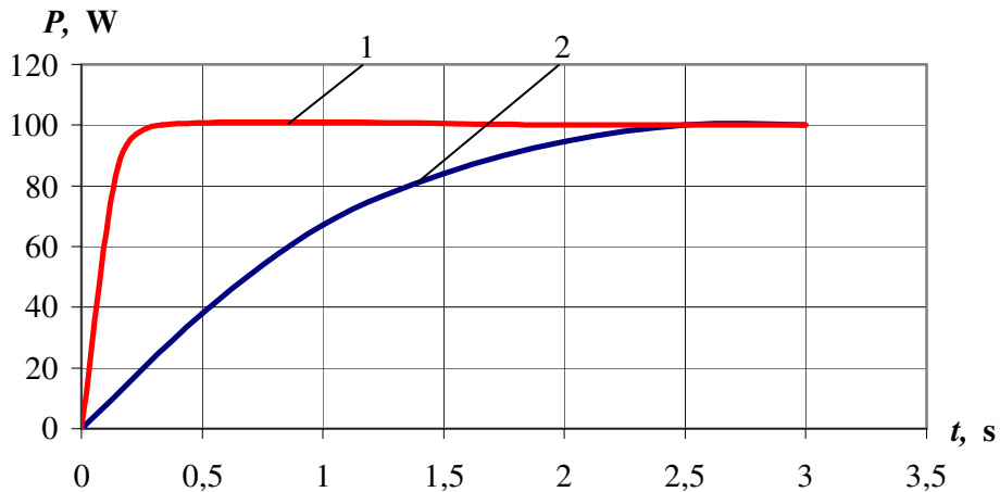
Рис. 2. Графічна залежність зміни споживання потужності P від часу роботи t для ламп розжарювання: 1 – звичайне вмикання; 2 – вмикання з диммером
